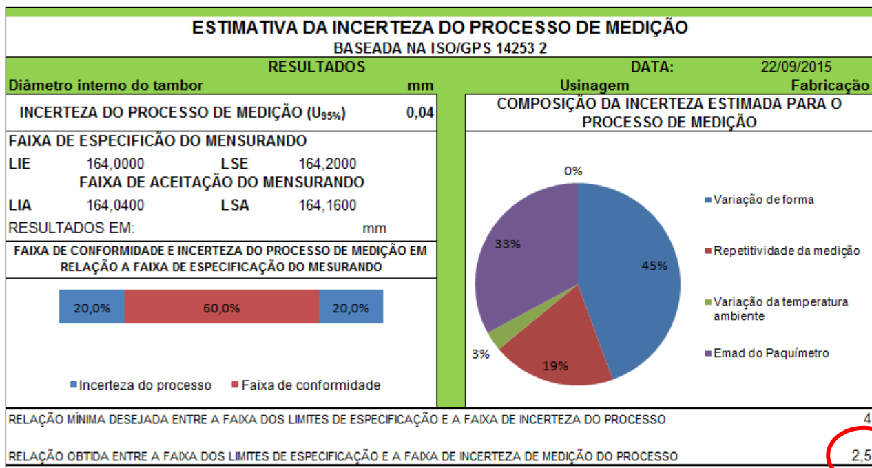
Quadro 3a - Análise dos resultados para o paquímetro digital
